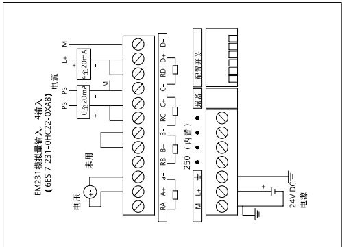
接线图
